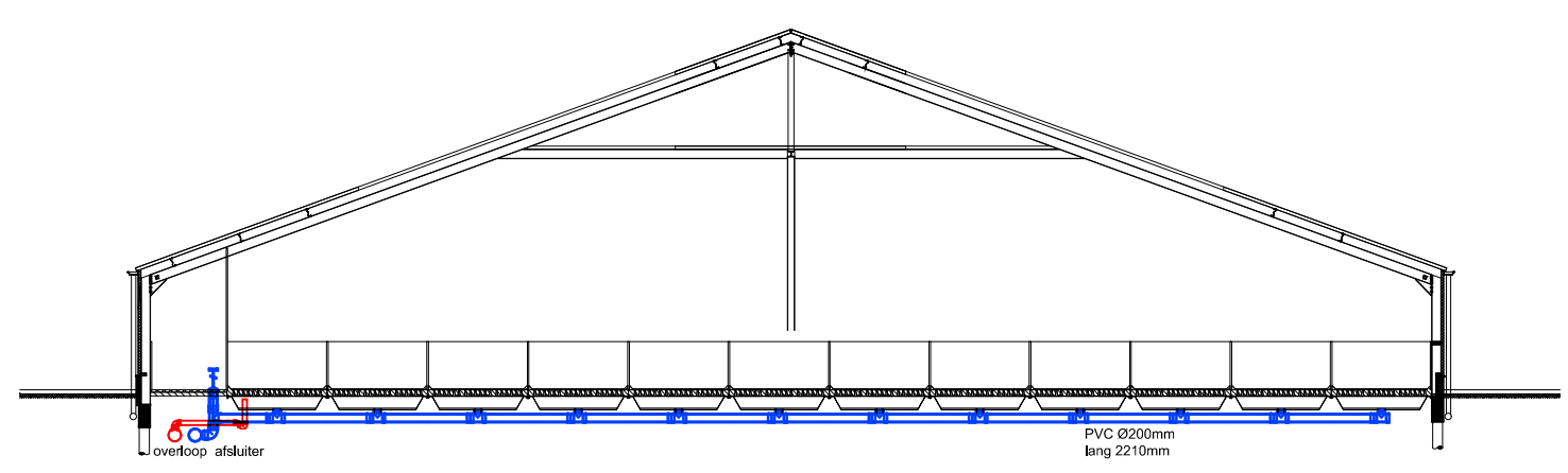
doorsnede A-A
