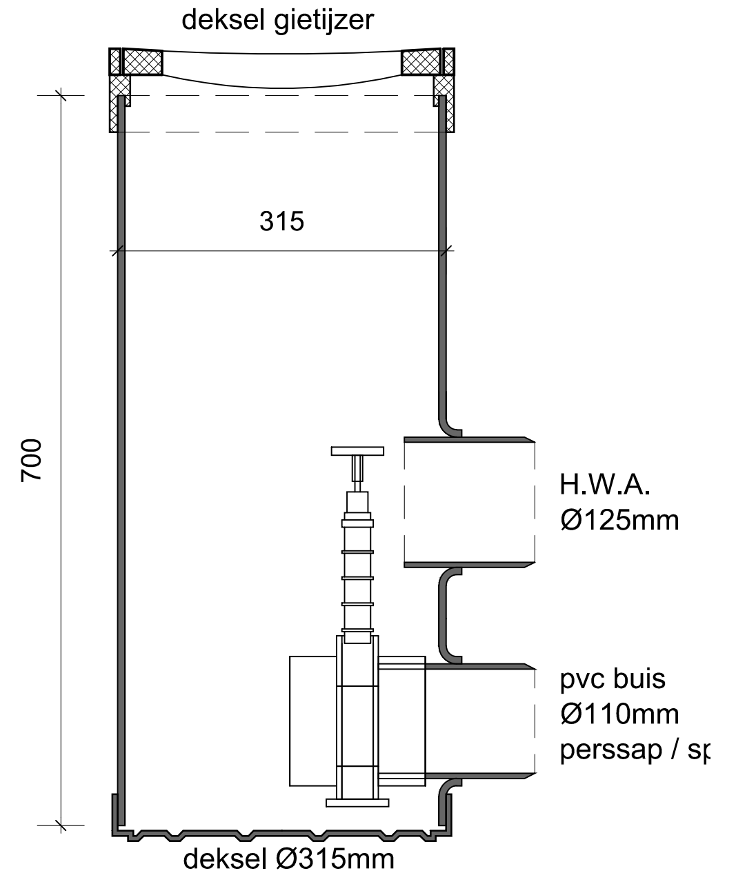
doorsnede
