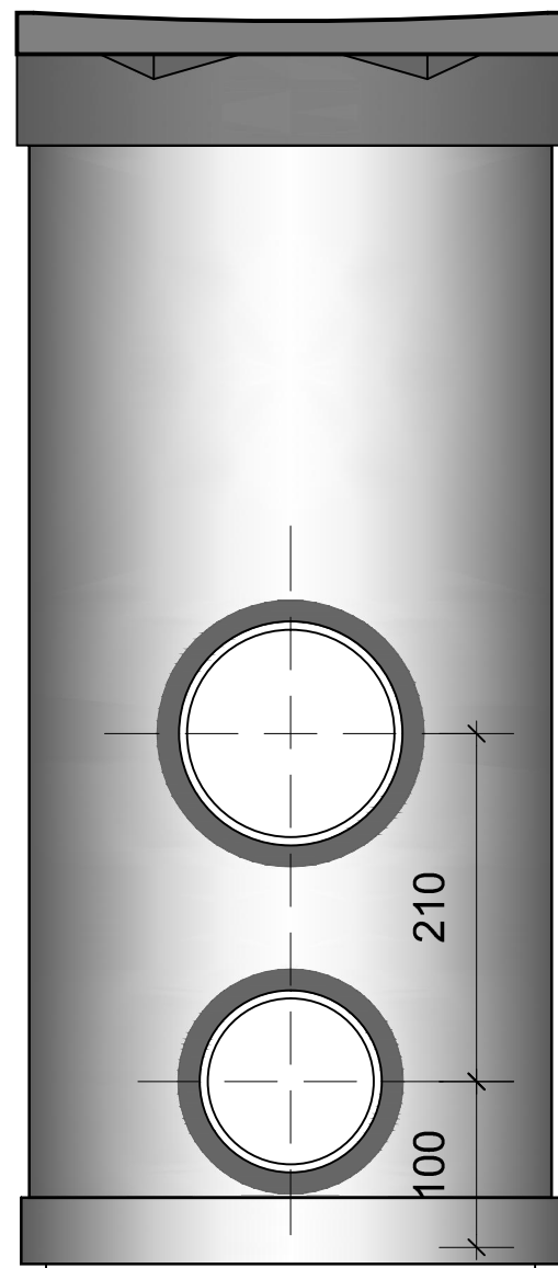
vooraanzicht
