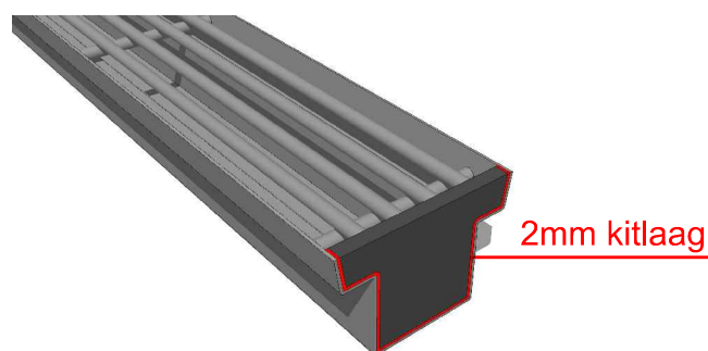
perspectief goot, afdichtingsplaat & rooster
