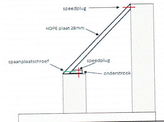
Doorsnede putplaat bij montage op muur
