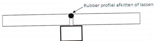
Doorsnede putplaat bij montage op putvloer
