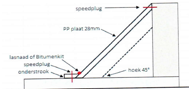
Doorsnede putplaat bij montage op muur
